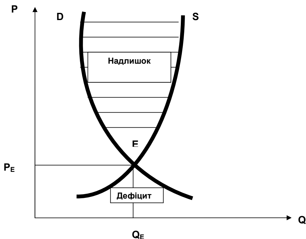
Рис. 4.1. Ринкова рівновага
